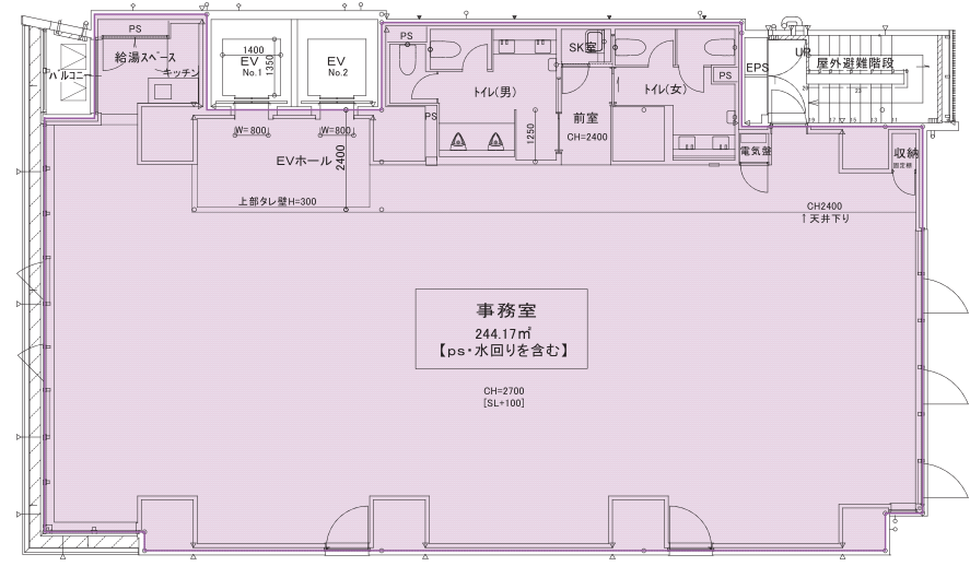
■基準階平面図(2~8階)
