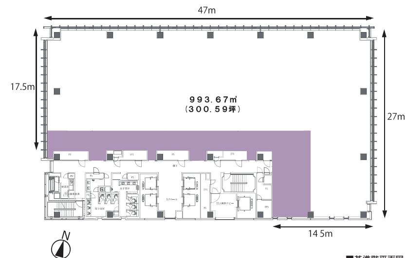
■基準階平面図
