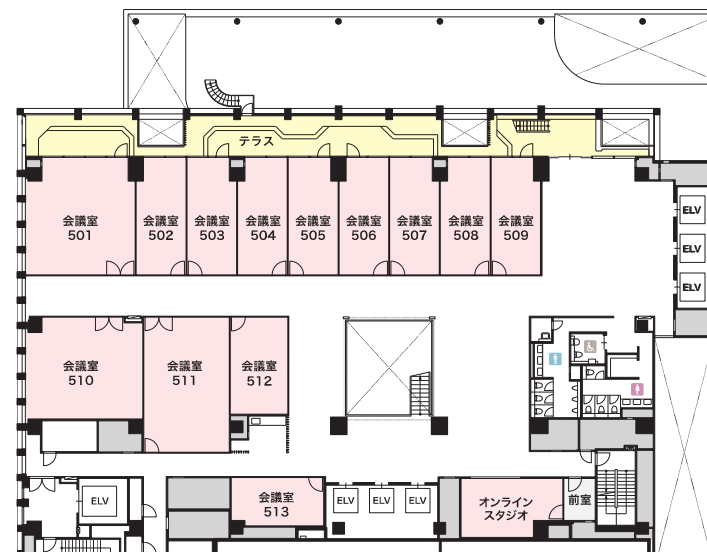
5階平面図
