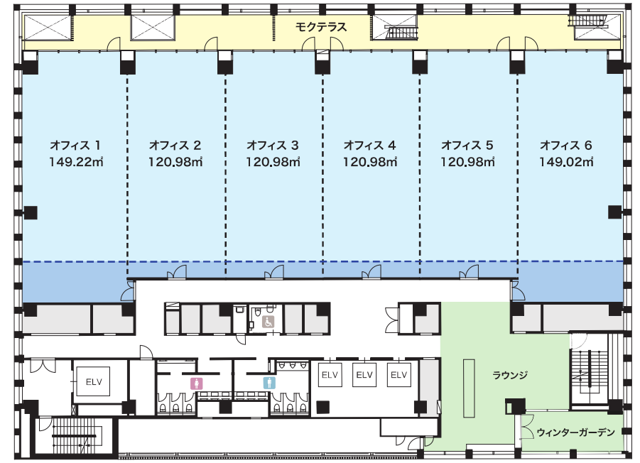
基準階 (10階)
